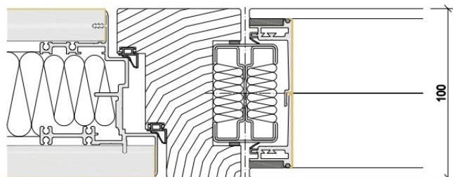
Volltür mit Holzblockrahmen
