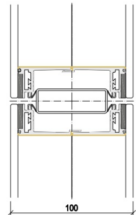
Höhenchnitt Natural Glazing Furnier
