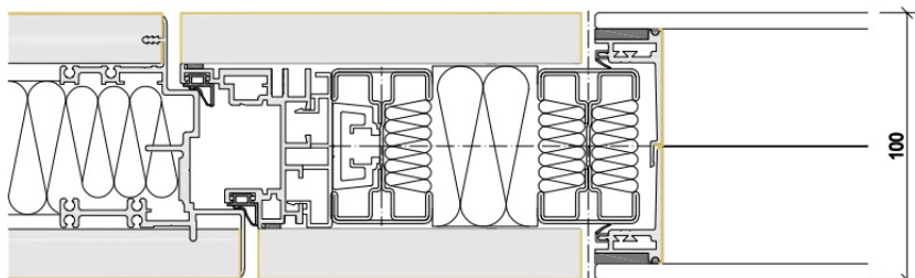
Volltür mit Aluminiumblock- rahmen als Portalelement
